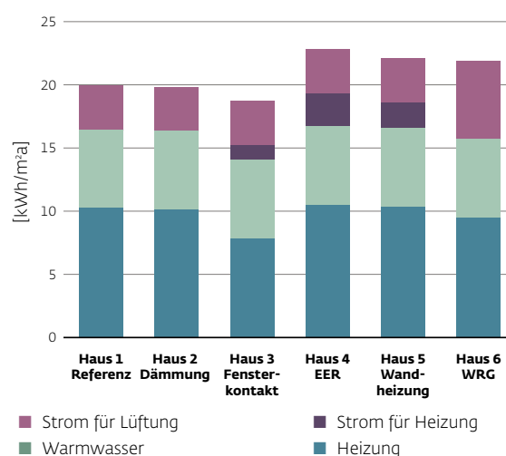
Primärenergiebedarf (bereinigt)
